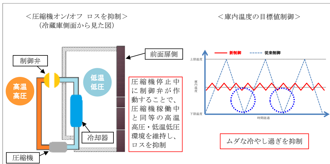
図 5 「NEW MICLOSS」 イメージ図
