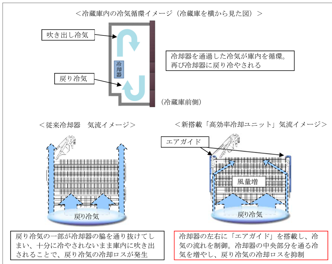
図 4 冷却器への戻り冷氣気流 イメージ図
