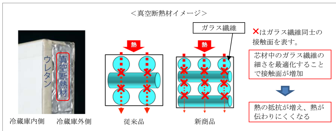
図3 高性能真空断熱材 イメージ図
