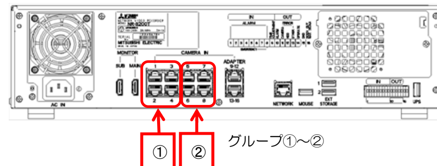
図2 NR-8200 のグループイメージ
