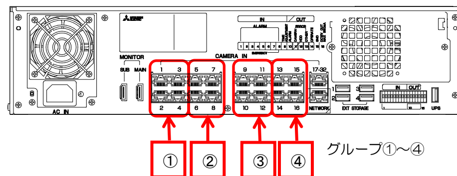
図1 NR-5000/5041/5080/5100のグループイメージ
