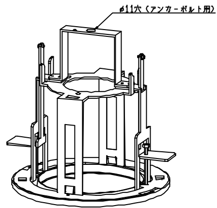
斜視図
