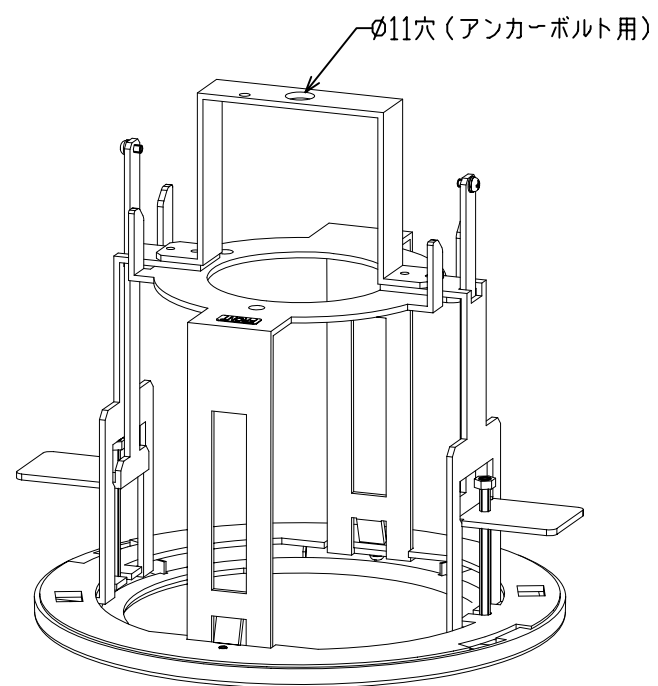
斜視図
