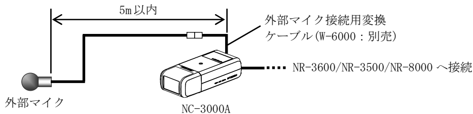
外部マイク使用時の接続
