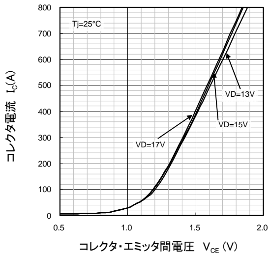
出力特性 (代表例)
