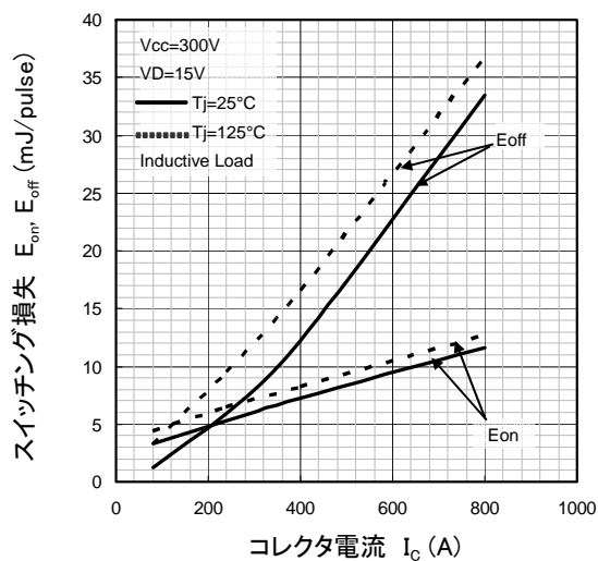
スイッチング損失特性 (代表例)
