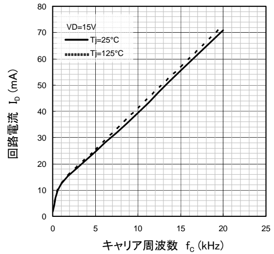
回路電流—キャリア周波数特性 (代表例)
