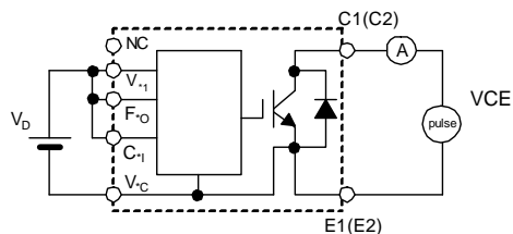
図 5. I_{CES} 試験
