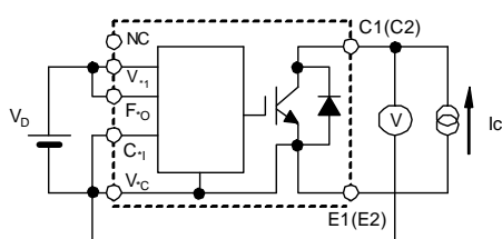
図 1. V_{OEsat} 試験
