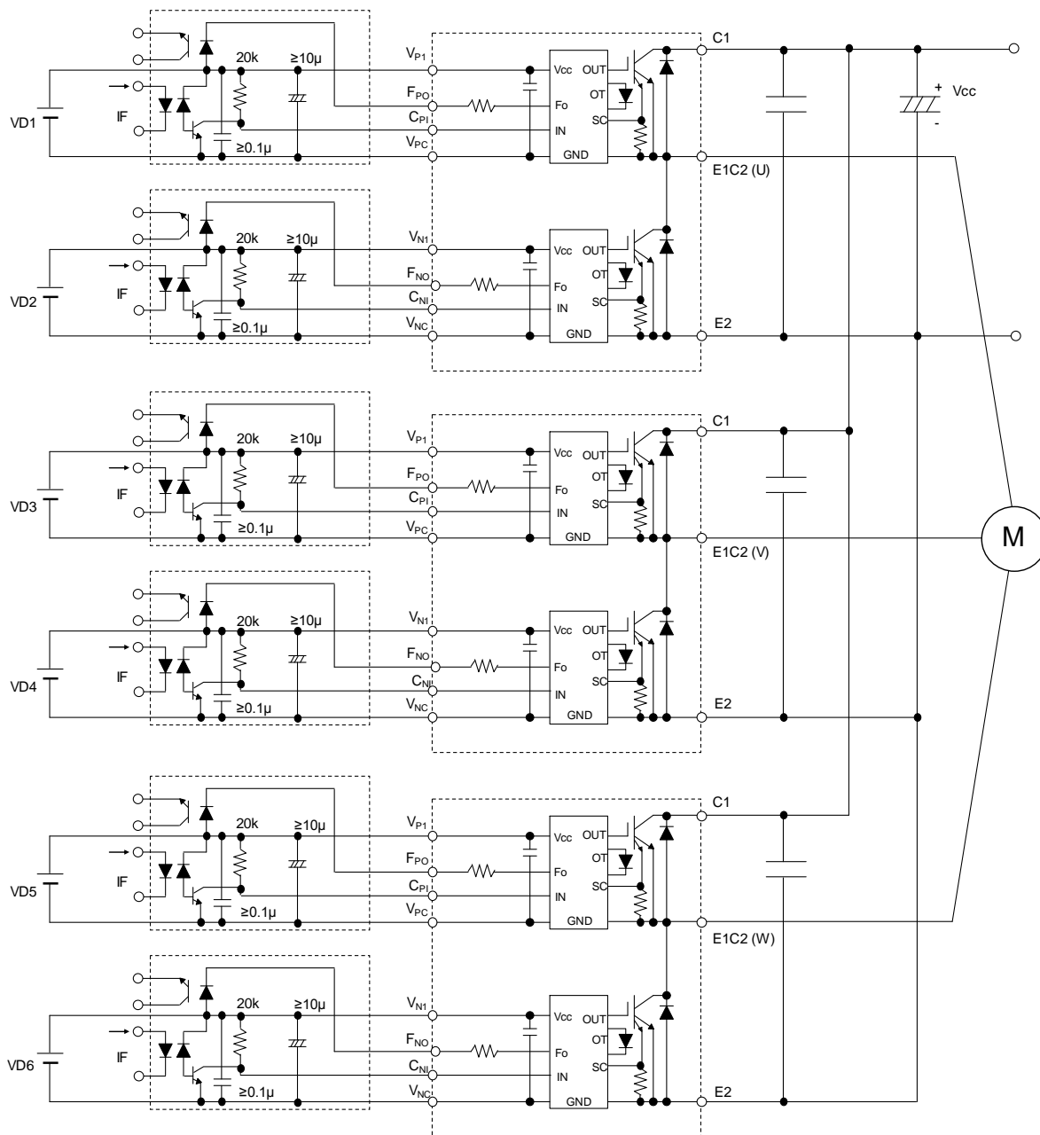
図 8. 応用回路例
