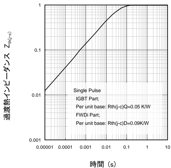
過渡熱インピーダンス特性 (代表例)
