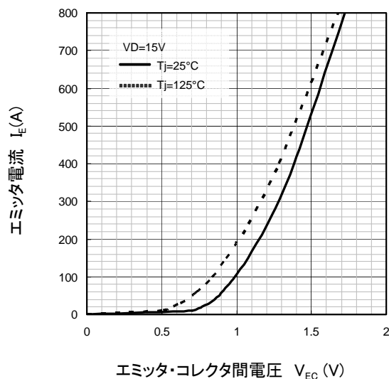
ダイオード部順方向特性 (代表例)
