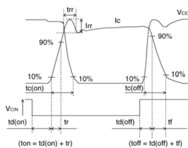
図 4. スイッチング時間試験波形
