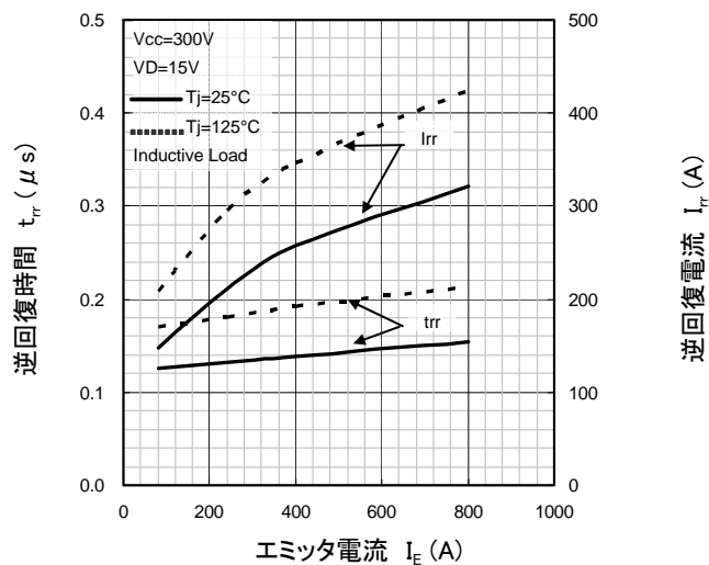
ダイオード部逆回復特性 (代表例)
