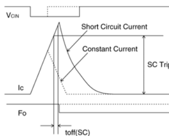
図 6. SC 試験波形
