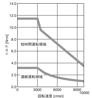
HK-MT103VW トルクアップ
