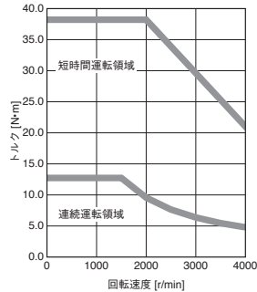
HK-ST202W トルクアップ
