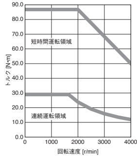
HK-ST502W トルクアップ
