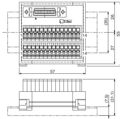
外形寸法図 (注1)
