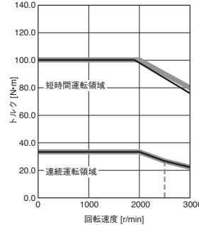
HK-ST7024W 標準トルク
