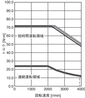
HK-ST5024W 標準トルク
