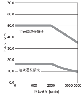
HK-ST352W 標準トルク
