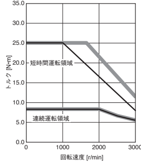
HK-ST172UW (注2) 標準トルク
