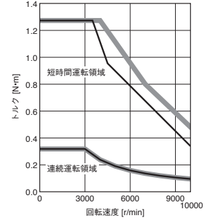
HK-MT13VW トルクアップ
