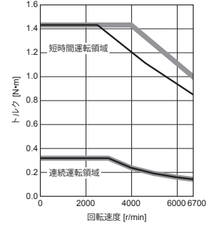
HK-KT13W トルクアップ
