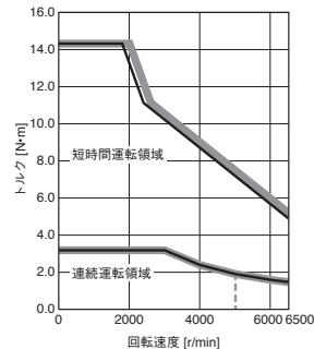
HK-KT1034W トルクアップ
