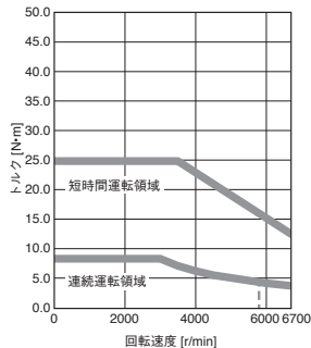
HK-ST353W 標準トルク
