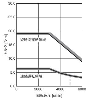
HK-KT2034W 標準トルク
