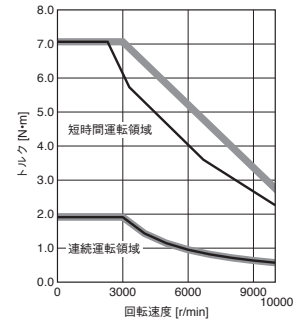
HK-MT63VW トルクアップ
