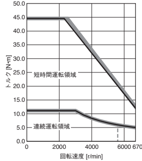
HK-ST3534W トルクアップ
