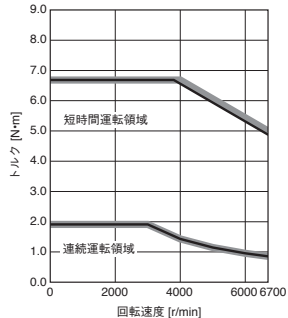
HK-KT634W 標準トルク
