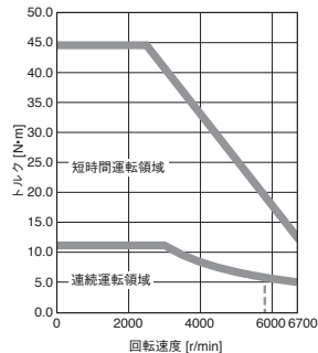
HK-ST353W トルクアップ
