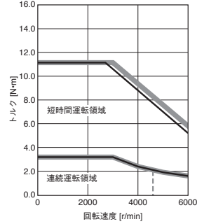
HK-KT1034UW 標準トルク
