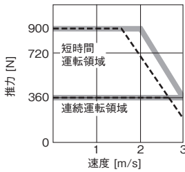
LM-H3P7B-48P-ASS0 (注1, 2, 3)
