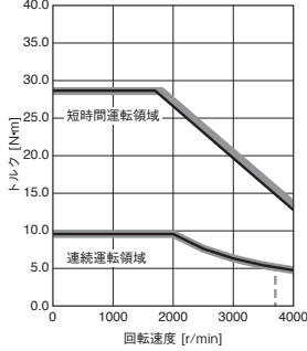
HK-ST2024W 標準トルク
