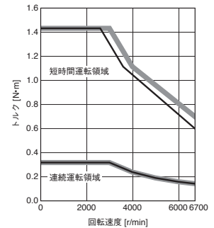
HK-KT13UW トルクアップ
