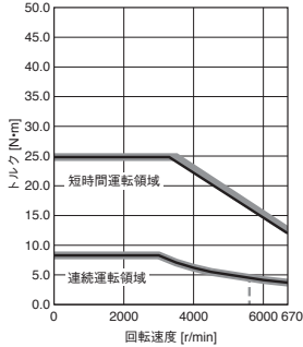
HK-ST3534W 標準トルク
