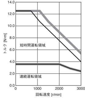
HK-ST7M2UW トルクアップ
