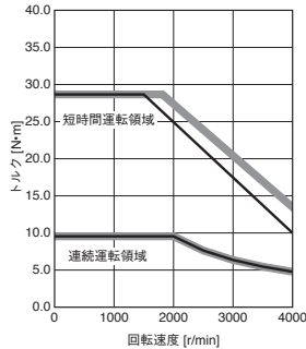
HK-ST202W (注2) 標準トルク
