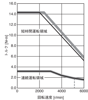
HK-KT103UW (注2) トルクアップ
