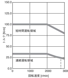
HK-ST702W 標準トルク
