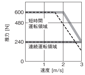
LM-H3P7A-24P-ASS0 (注1, 2, 3)
