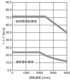
HK-ST502W 標準トルク
