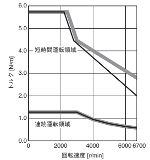
HK-KT43W トルクアップ
