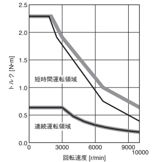
HK-MT23VW トルクアップ
