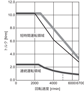
HK-KT63UW トルクアップ
