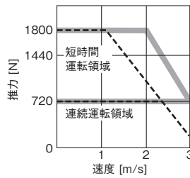
LM-H3P7C-72P-ASS0 (注1, 2, 3)
