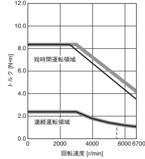
HK-KT7M3UW 標準トルク
