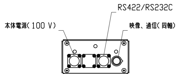
A矢视图(コネクタ配置)
