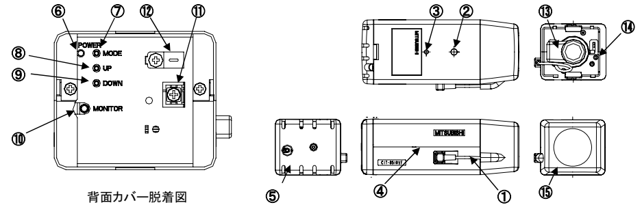
背面カバー脱着図
