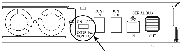
増設 HDD ユニット(DX-ZD6)の EXTERNAL SW を“ON”にする。
