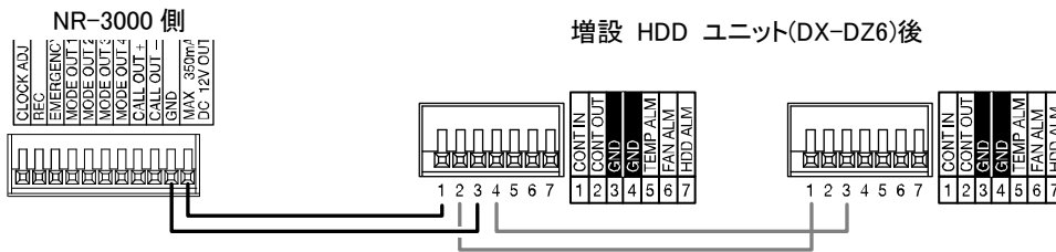
増設 HDD ユニット(DX-ZD6)の EXTERNAL SW を“ON”にする。
