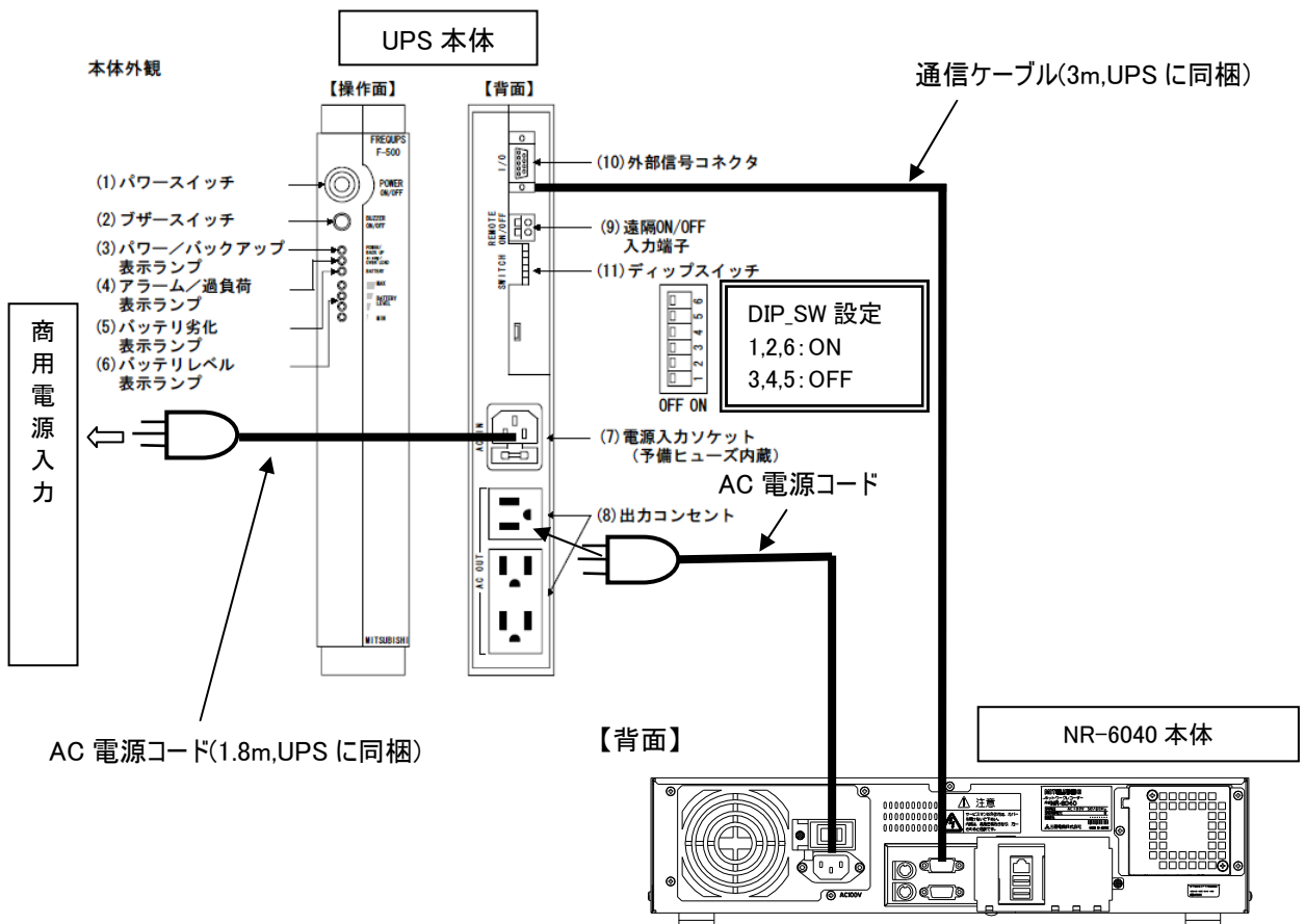
付図 1 本機(NR-6040)とUPSの設定及び接続
