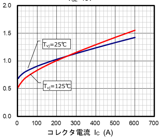
コレクタ・エミッタ間飽和電圧測定 (代表例：チップ)
