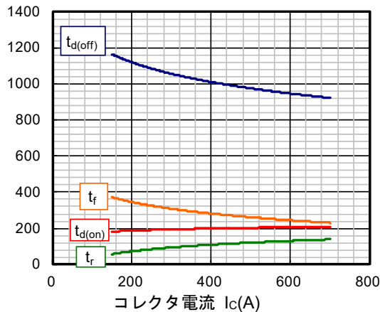
スイッチング特性 (代表例)
