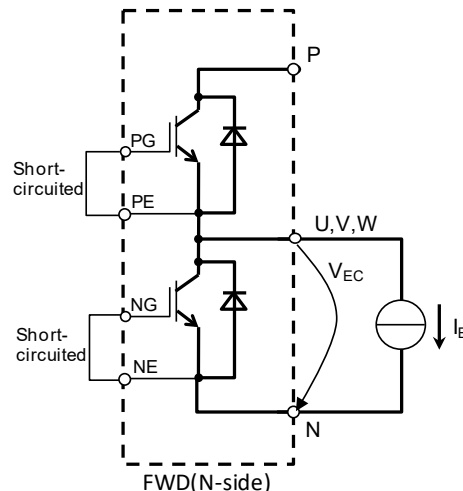
V_{EC} 測定回路図(主端子間)
