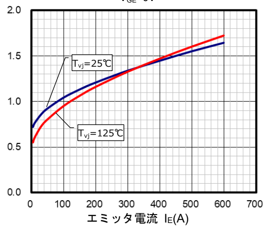
ダイオード部順方向特性 (代表例：チップ)
