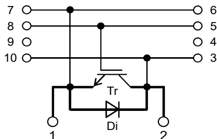
内部接続図
