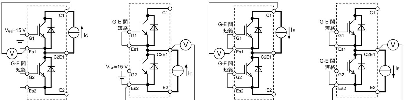
V_{CEsat} 試験回路
