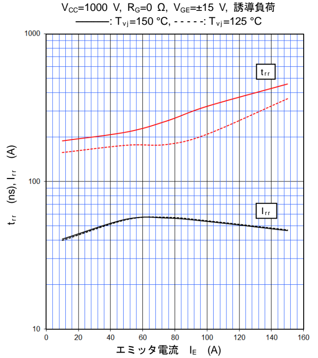
フリーホイールダイオード逆回復特性 (代表例)
