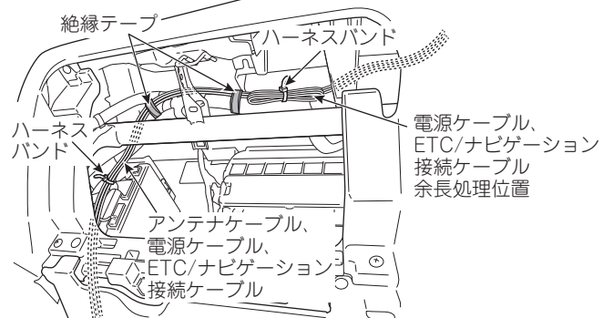
＜グローブボックス裏側＞
