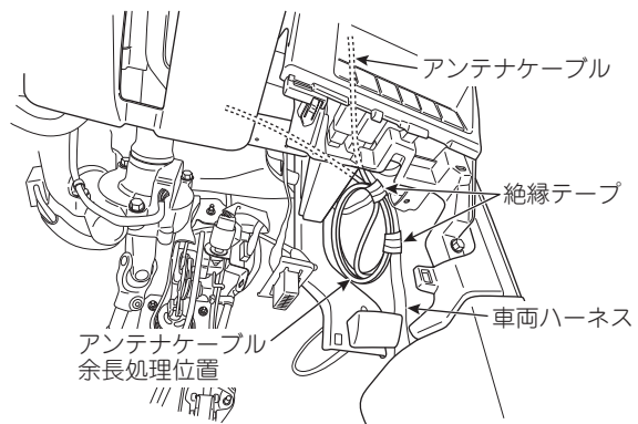
＜インパネアンダートレー裏側(ステアリング右下)＞
