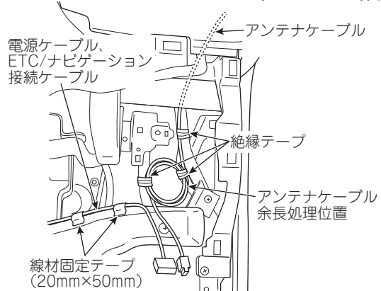
＜インストールロアパネル(運転席側)裏側 (ステアリング右下)＞
