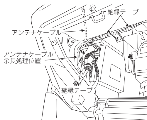
＜グローブボックス裏側＞
