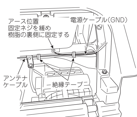
＜グローブボックス裏側 アース位置＞
