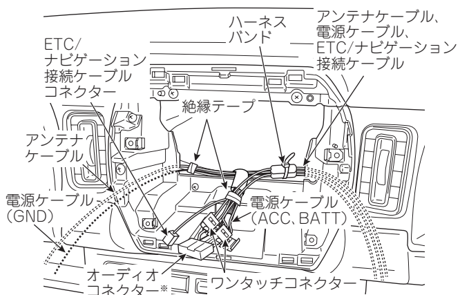
＜オーディオユニット裏側＞
