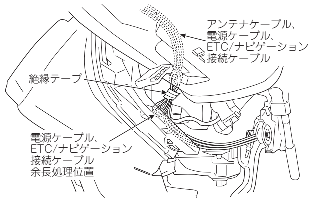
＜インパネアンダートレー裏側(ステアリング左下)＞
