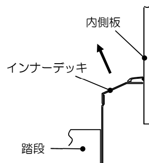
インナーデッキ取り外し
