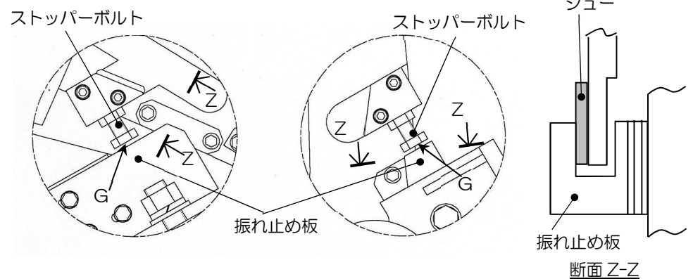
7-3-2 の C 部詳細
