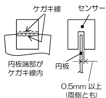
センサーと円板の関係
