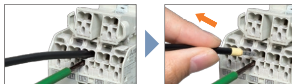
工具を工具挿入口の奥まで差し込む
