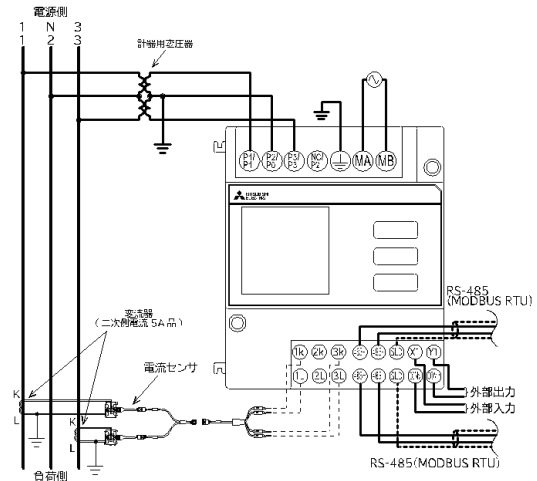
【単相3線式／三相3線式（2CT）（高圧回路）】
