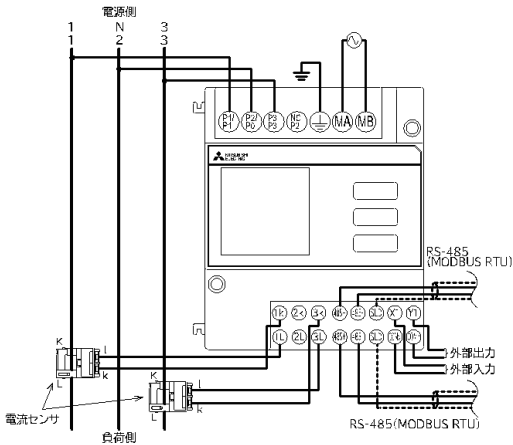
【単相3線式／三相3線式（2CT）（低圧回路）】
