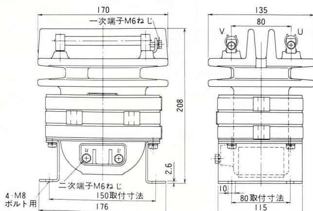
図1. EMT-K形
