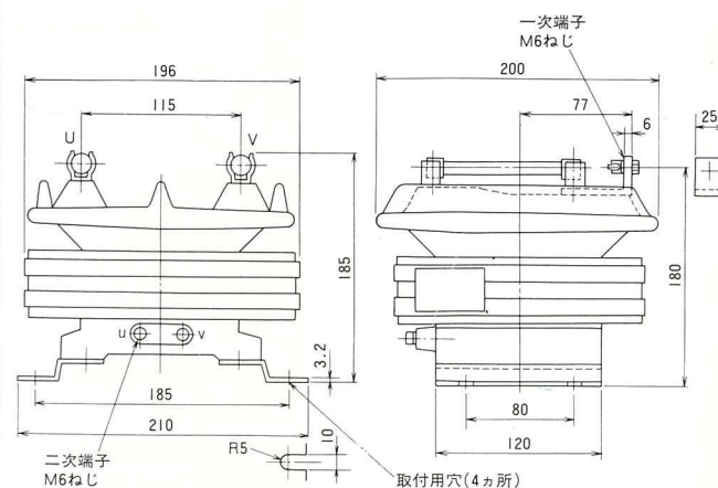
図2. EMT-BA形
