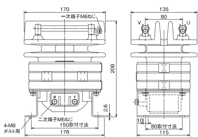
図 1. EMT-K 形
