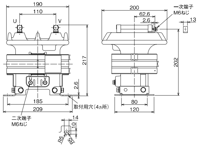
図 2. EMT-BB 形
