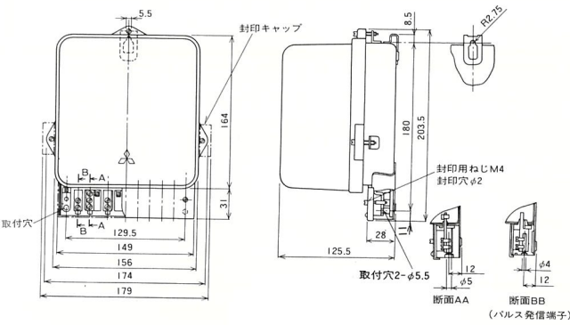
M2B-K11形(120A)
