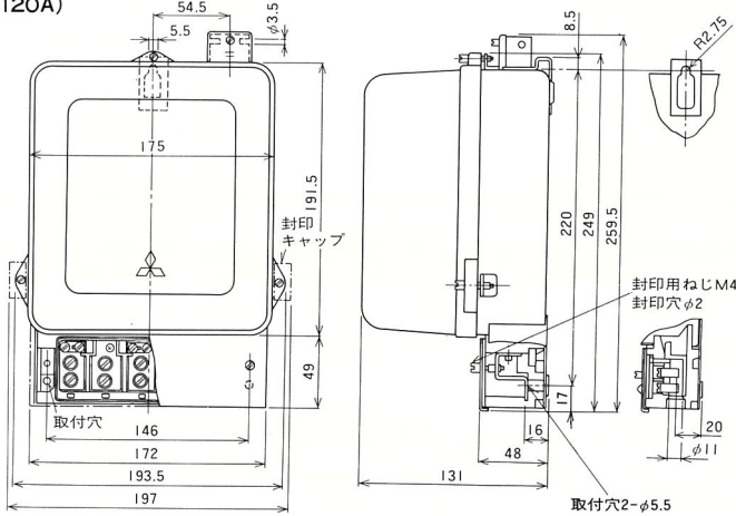
M2B-K11形(120A)
