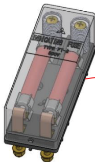
図 1. 【変更前】外観及び変更箇所 (FT-2 形)
