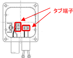
過励磁電源装置(例:200V 屋内形)
