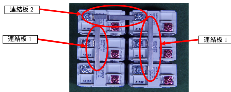
図 連結板使用箇所
