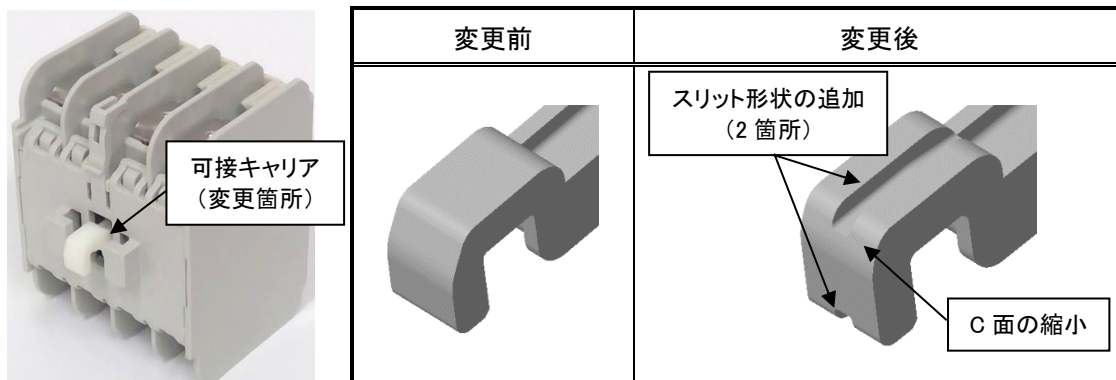
図. 製品外観写真 (代表機種 UT-AX4)
