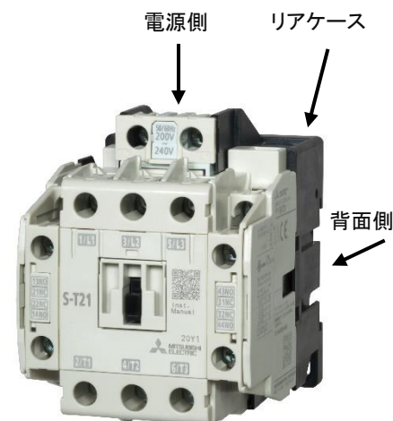
図 1: 製品外観(S-T21)
