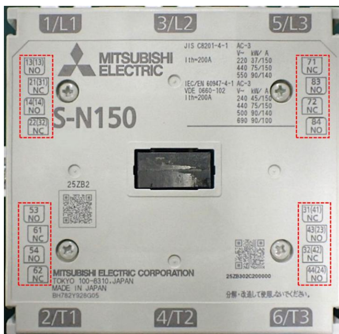
図 1. 端子番号表示(代表機種:S-N150 形電磁接触器)
