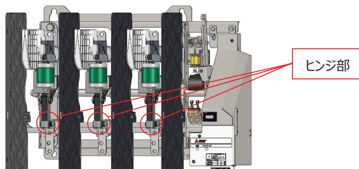
図 1. 外観及び変更箇所 (代表例: TES-GA 形)
