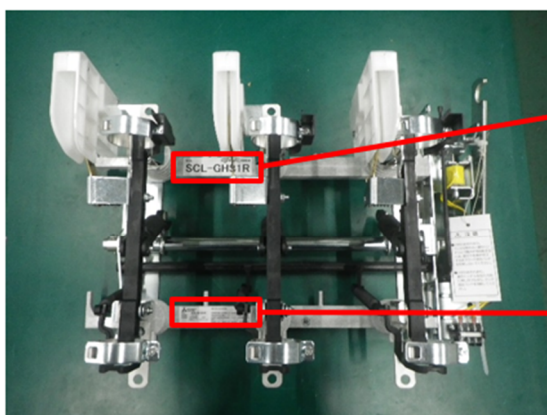
図1.LBS外観
