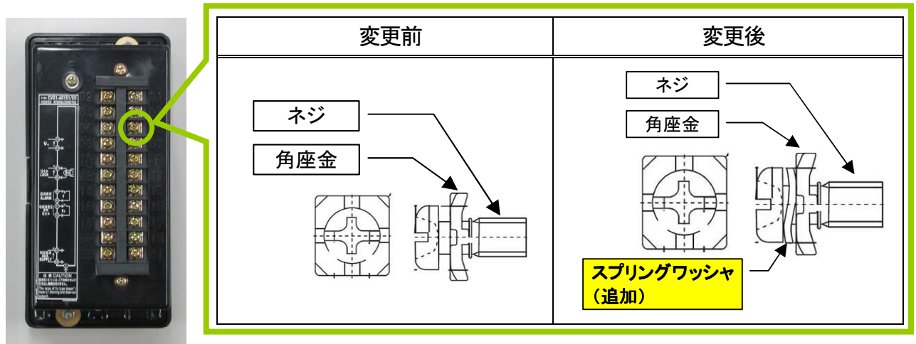
端子台
