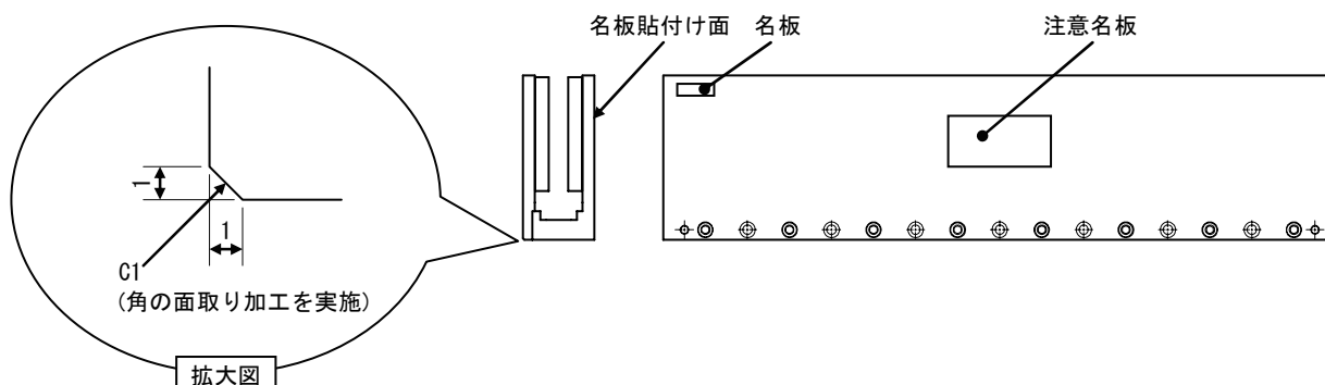
図1. 面取り箇所 (LM-U2S20-480-2SS0の例)
