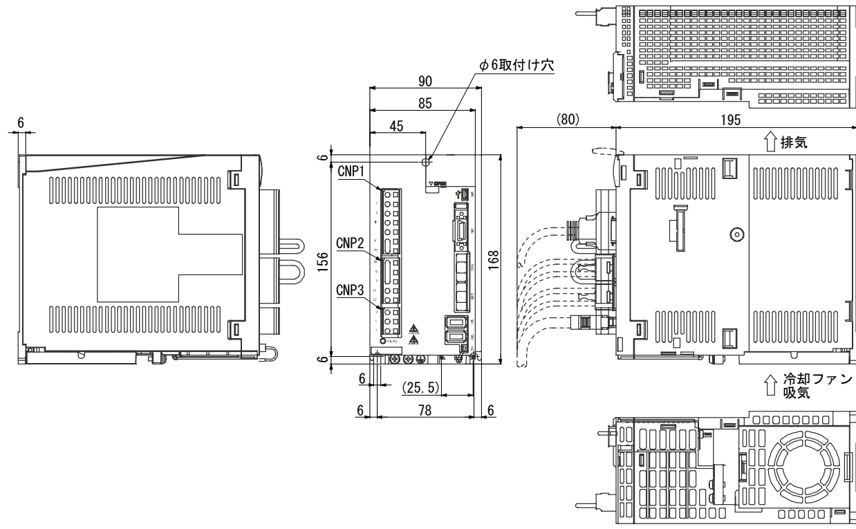
MR-J3-200BN-RJ006外形図
