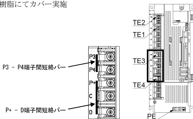
図1. MR-J4-500_外形図 (正面カバーを開けた状態)
