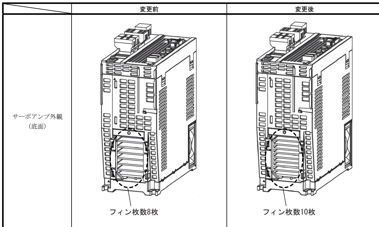
図1. サーボアンプ内部放熱フィン形状
