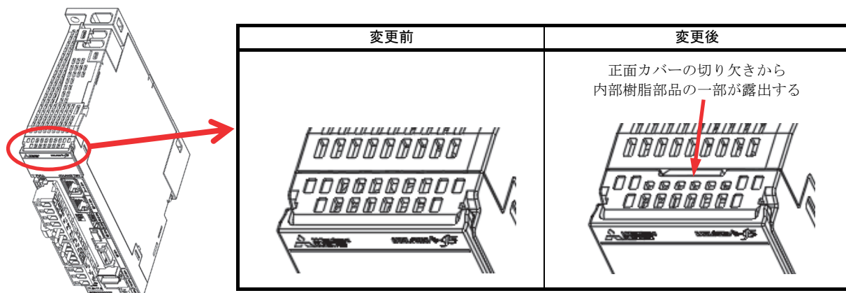
図1. 正面カバーと内部樹脂部品の変更
