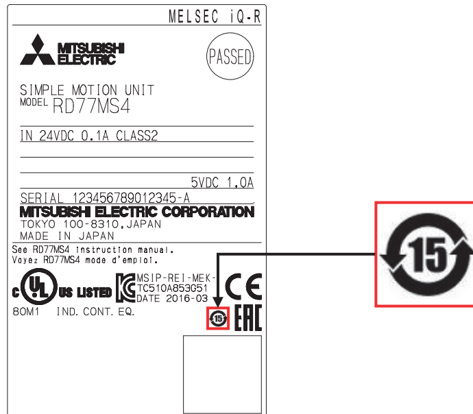
図1. 表示例 (RD77MS4)
