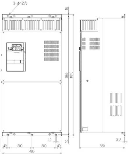
■FR-A740-160K, 185K
