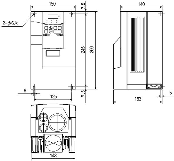
■FR-V520-1.5K, 2.2K
