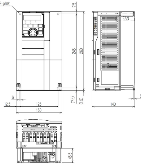
■FR-A820-2.2K, 3.7K
