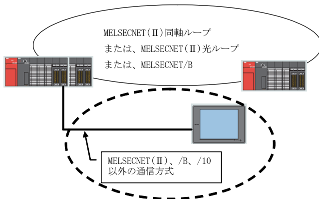
図5-2 空きスロットのあるシーケンサに通信ユニット増設し GOTとシーケンサを接続する置き換え構成例
