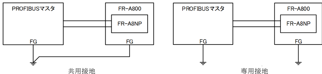
図 2 共用接地／専用接地
