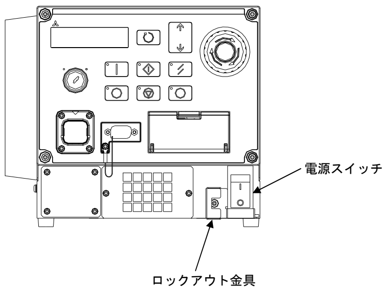
図1. コントローラ正面図
