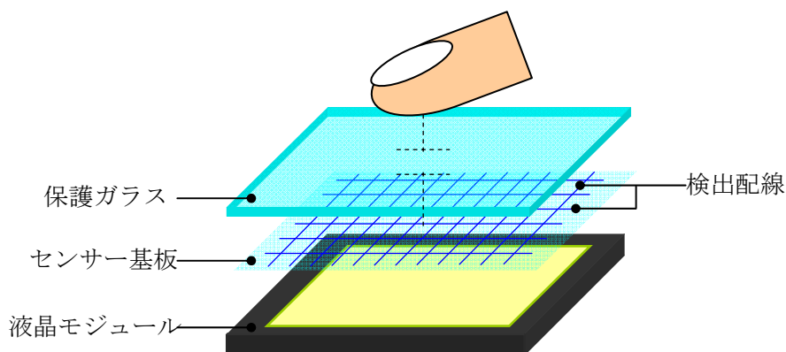
【投影型静電容量方式タッチパネル搭載液晶モジュール概略図】
