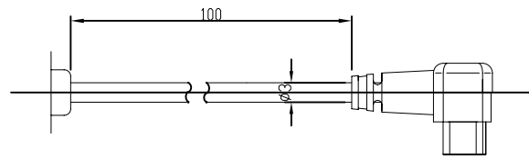
アイリスコントロールケーブル IRIS CONTROL CABLE (CONNECTOR: 4-PIN PLUG)
