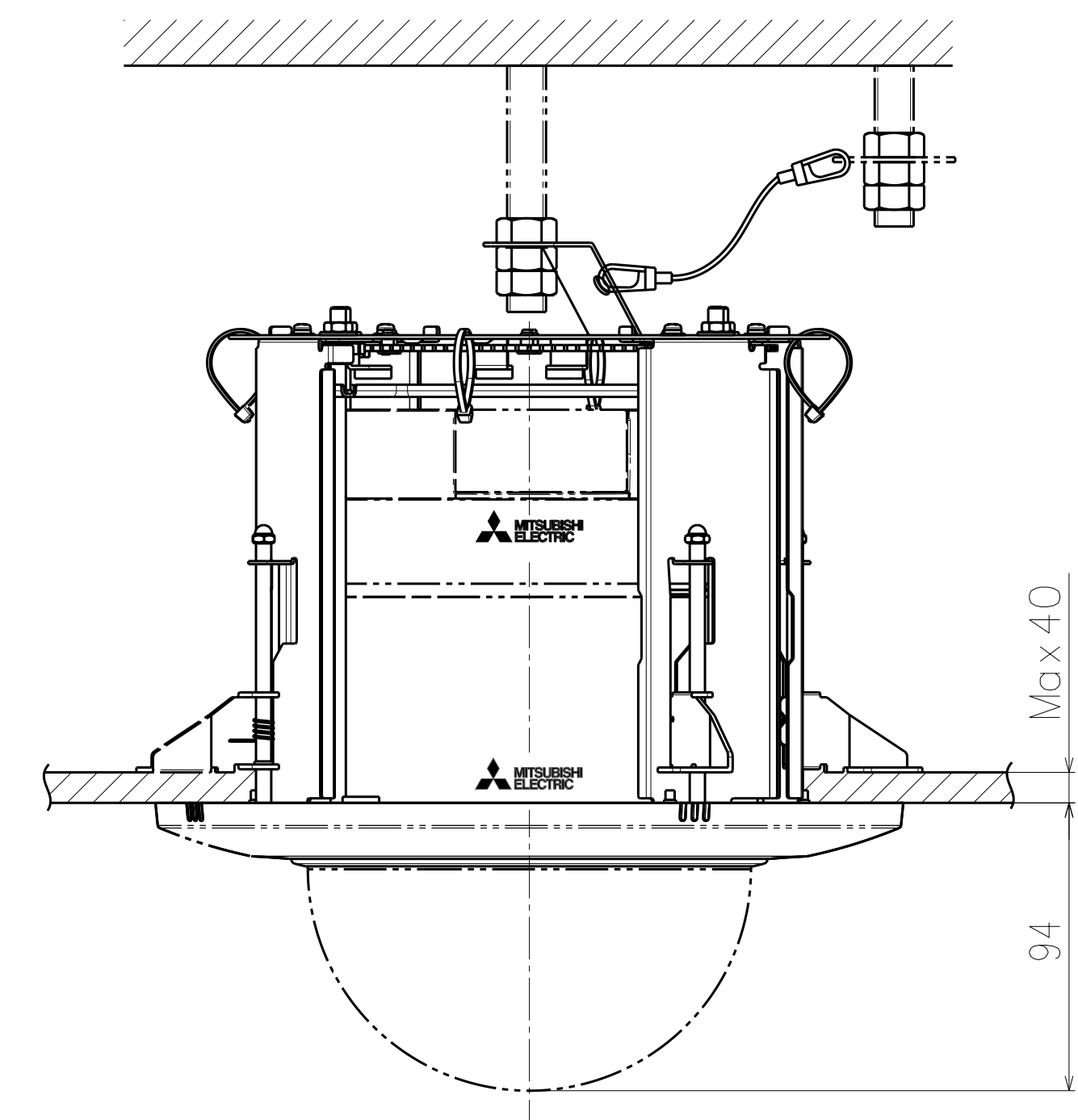
NC-9520とK-9971との組み合わせ図
