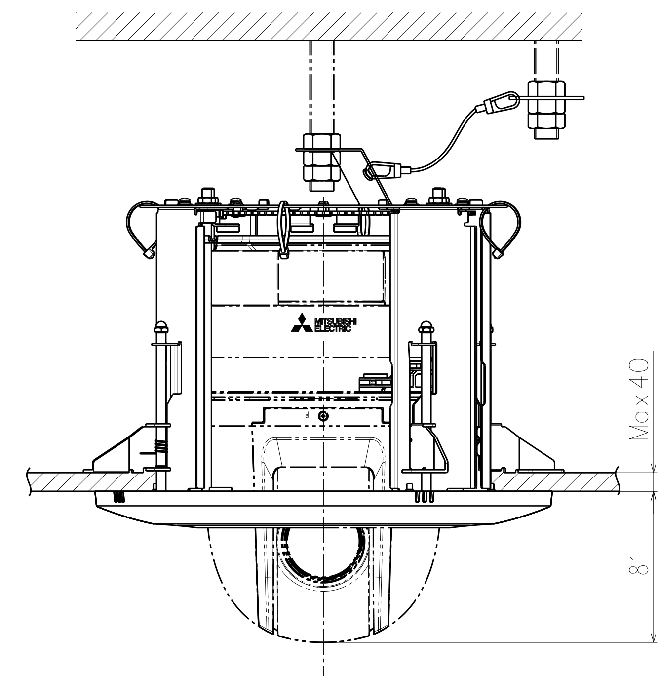
NC-9520との組み合わせ図
