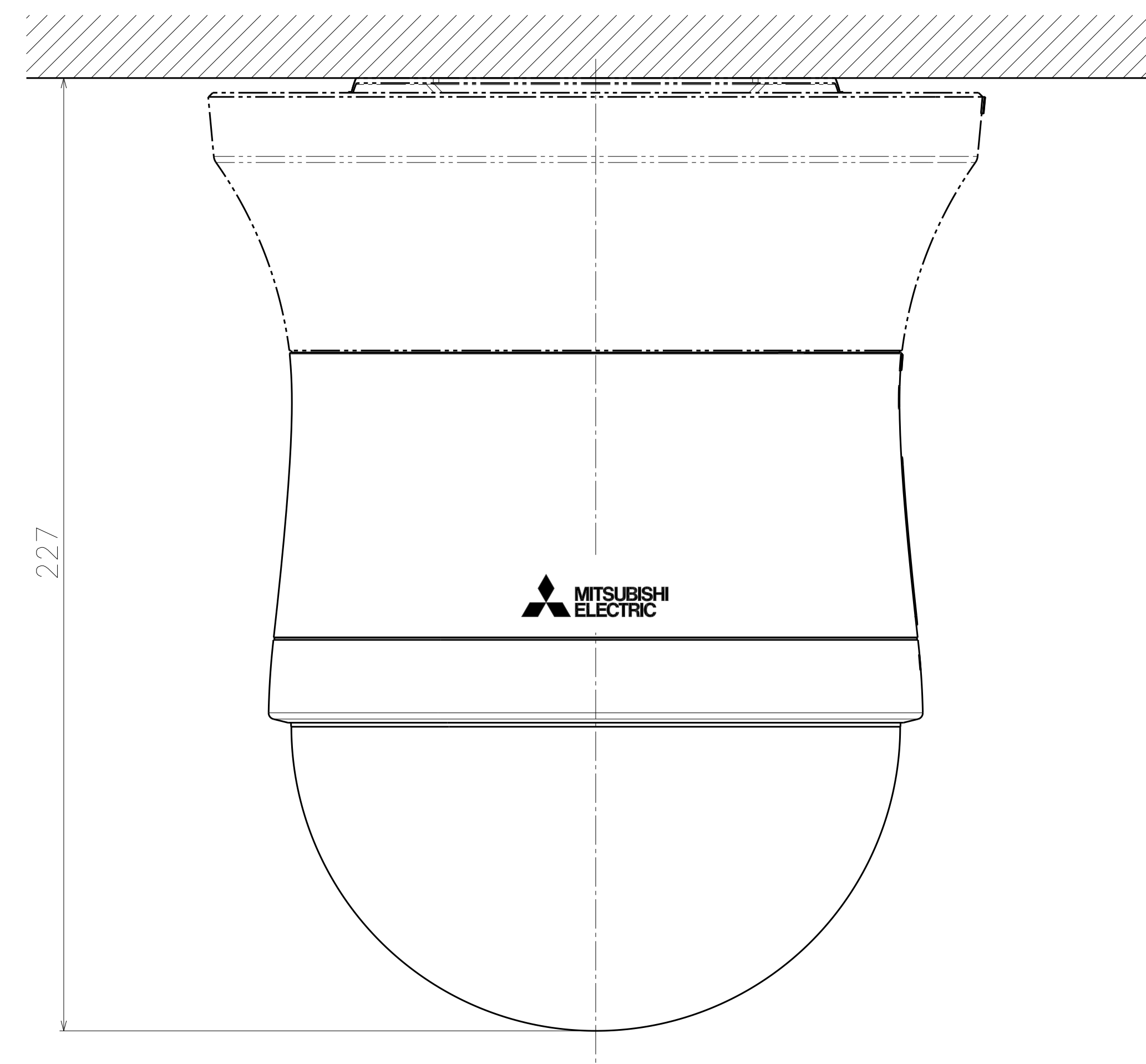
NC-9520との組み合わせ図
