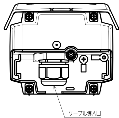
矢視A カバーをはずした状態
