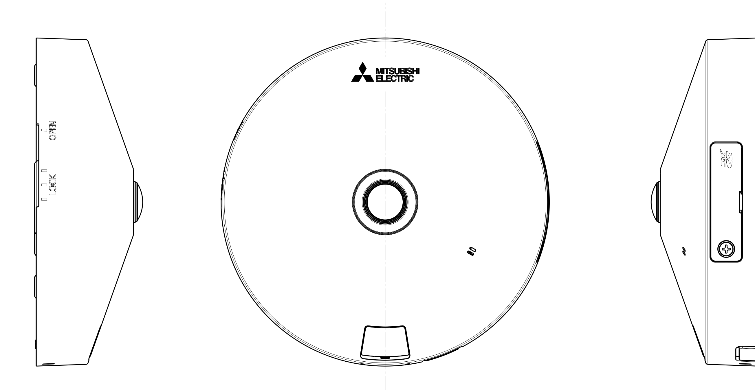
SDスロットカバーを外した図
