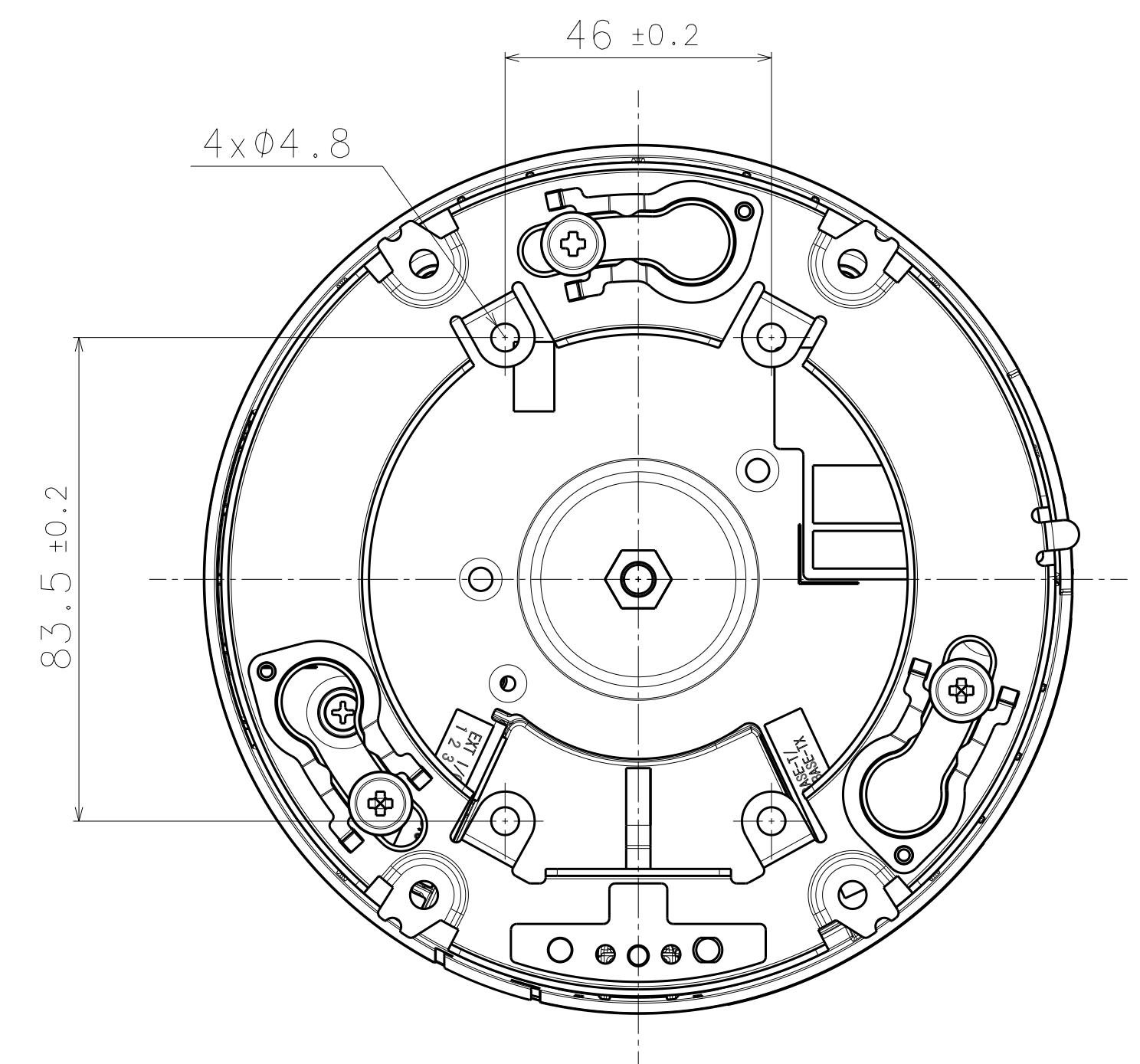
アタッチメントプレートを付けた図
