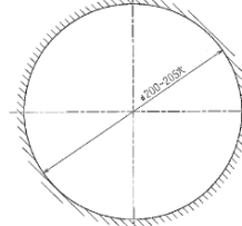
取付け面加工寸法図
