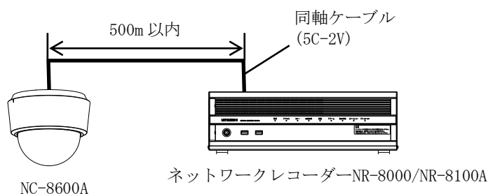
I. ネットワークレコーダーから電源供給する場合の接続構成例
