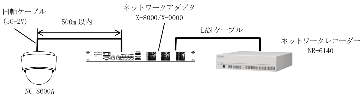
II. ネットワークアダプタから電源供給する場合の接続構成例 (DG II モード)
